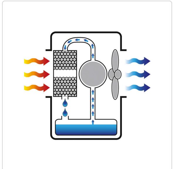
Diagramma di raffreddamento evaporativo Master
