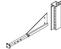
STAFFA PROLUNGABILE Adjustable support Support extensible Verlängerungsbügel
