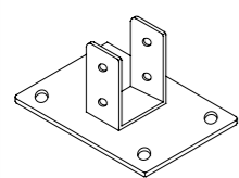
PIASTRA DI BASE MONTANTE BIFRONTA Base plates double sided uprights Plaque de base montant bifrontal Grundplatte zweiseitige Träger
