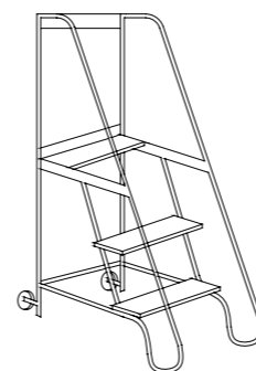
SCALA SGABELLO ACCIAIO INOX E ALLUMINIO Aluminum and stainless stool stairs Échelle plate-forme individuel en acier et aluminium Stahlblech und Aluminium Podestleiter
