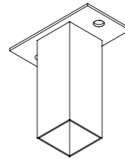
INNESTO TUBOLARE FISSAGGIO MONTANTE/SOFFITTO Tubing connection double sided uprights Manchon à tube Rohranschluß zweiseitige Träger
