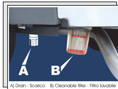
A) Drain - Scarico B) Cleanable filter - Filtro lavabile
